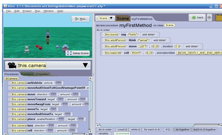
Рис. 2. Описание обработчика события для объекта
